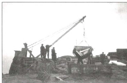
El difícil acceso al Islote llevó a la construcción de un aparejo mecánico para el desembarco de cargas.
